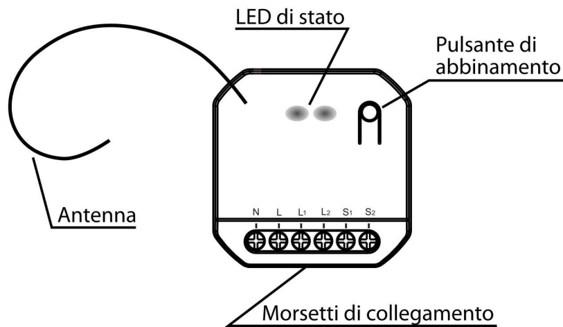
Il vostro Attuatore doppio smart Wi-Fi 9325
